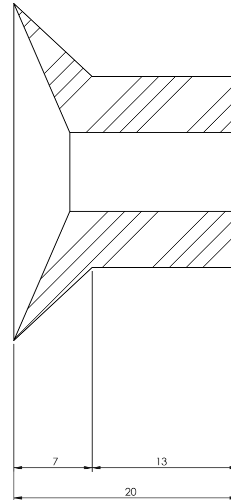
SEZIONE D-D
